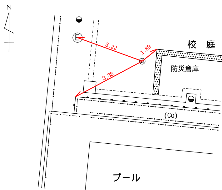
詳細図
