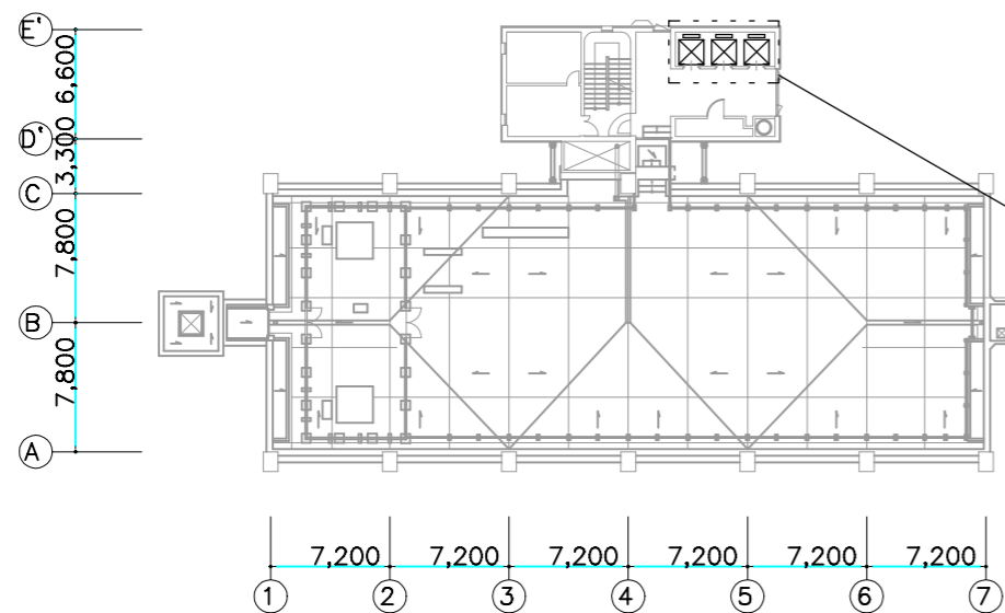
塔屋1階平面図 1/500
