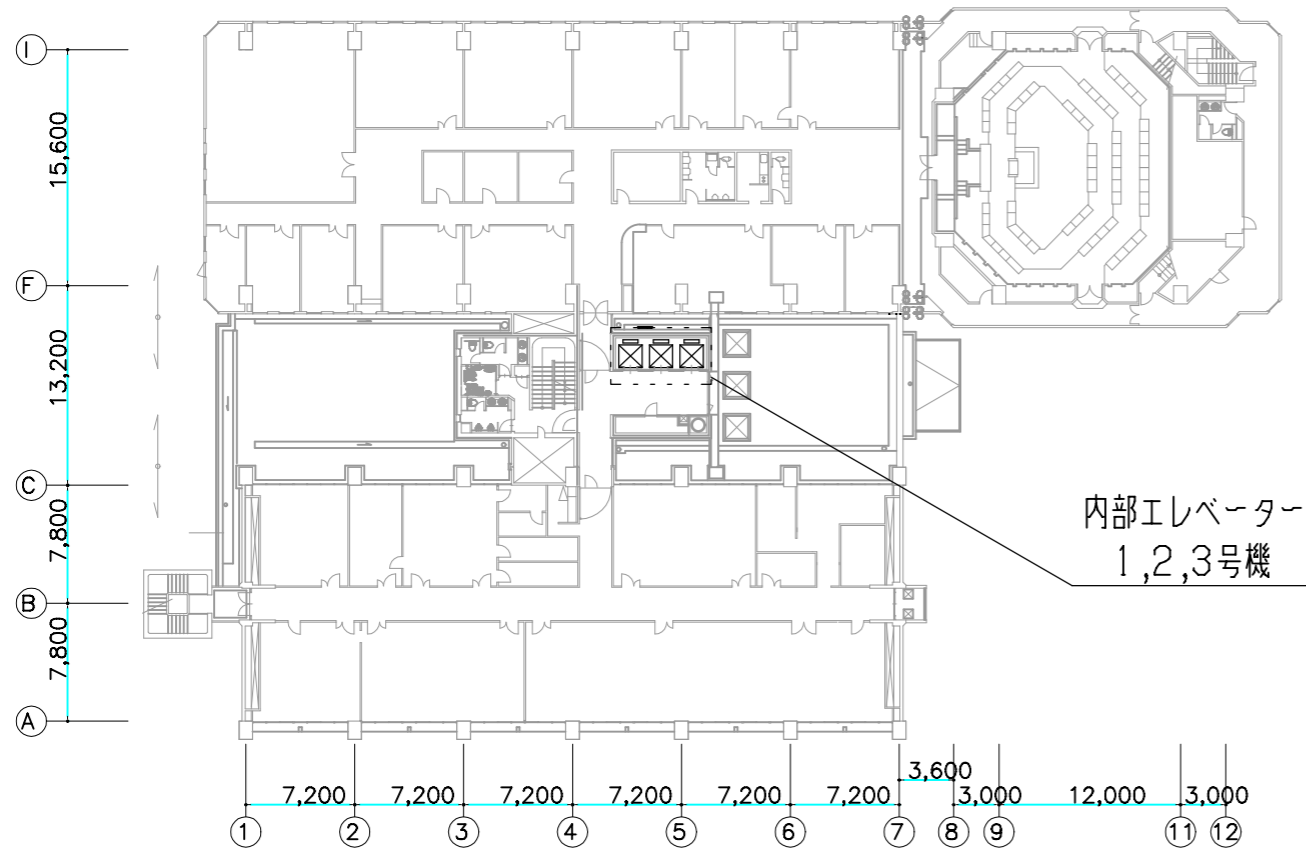
4階平面図 1/500
