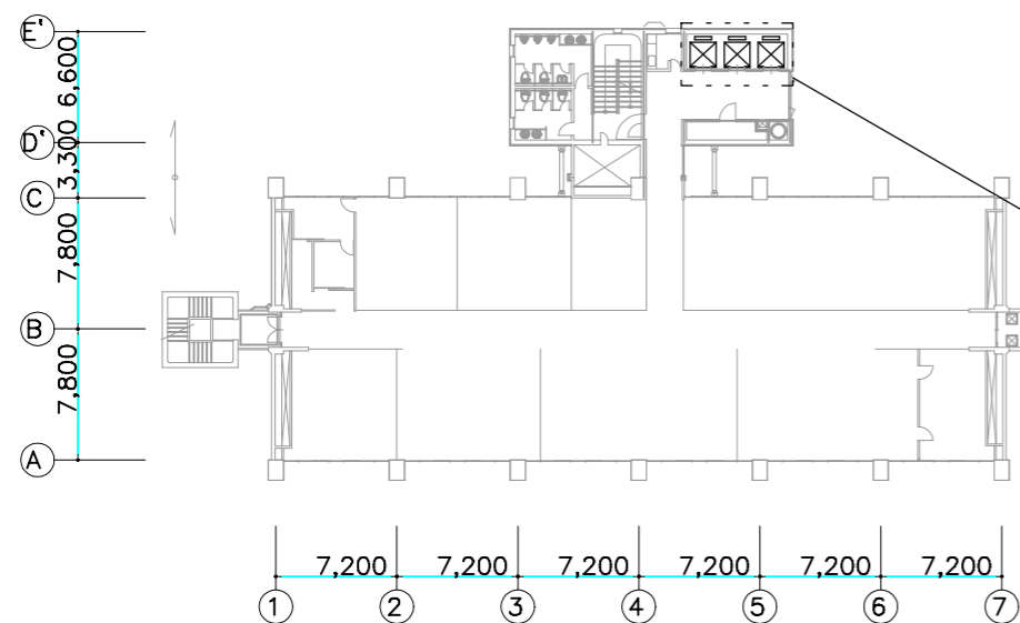
8階平面図 1/500
