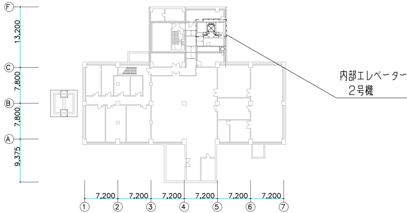
B階平面図 1/500
