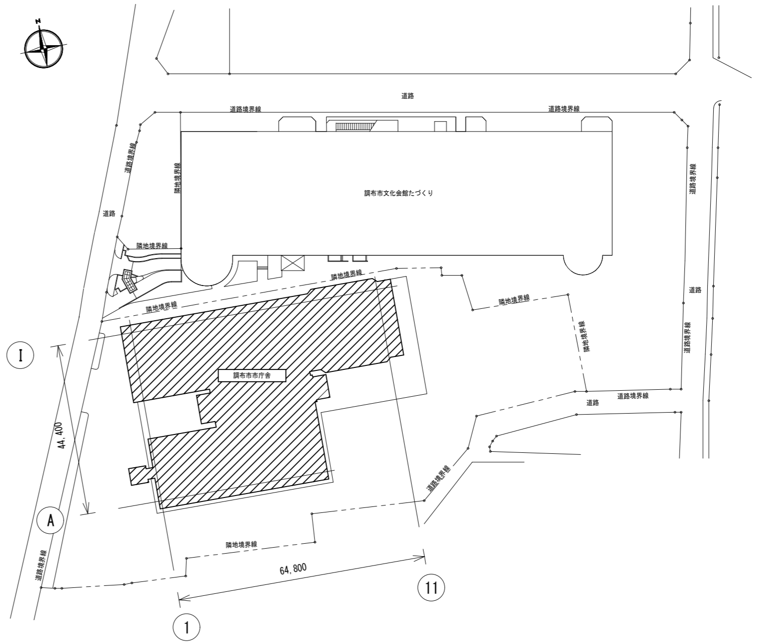
配置図 S=1/1000
