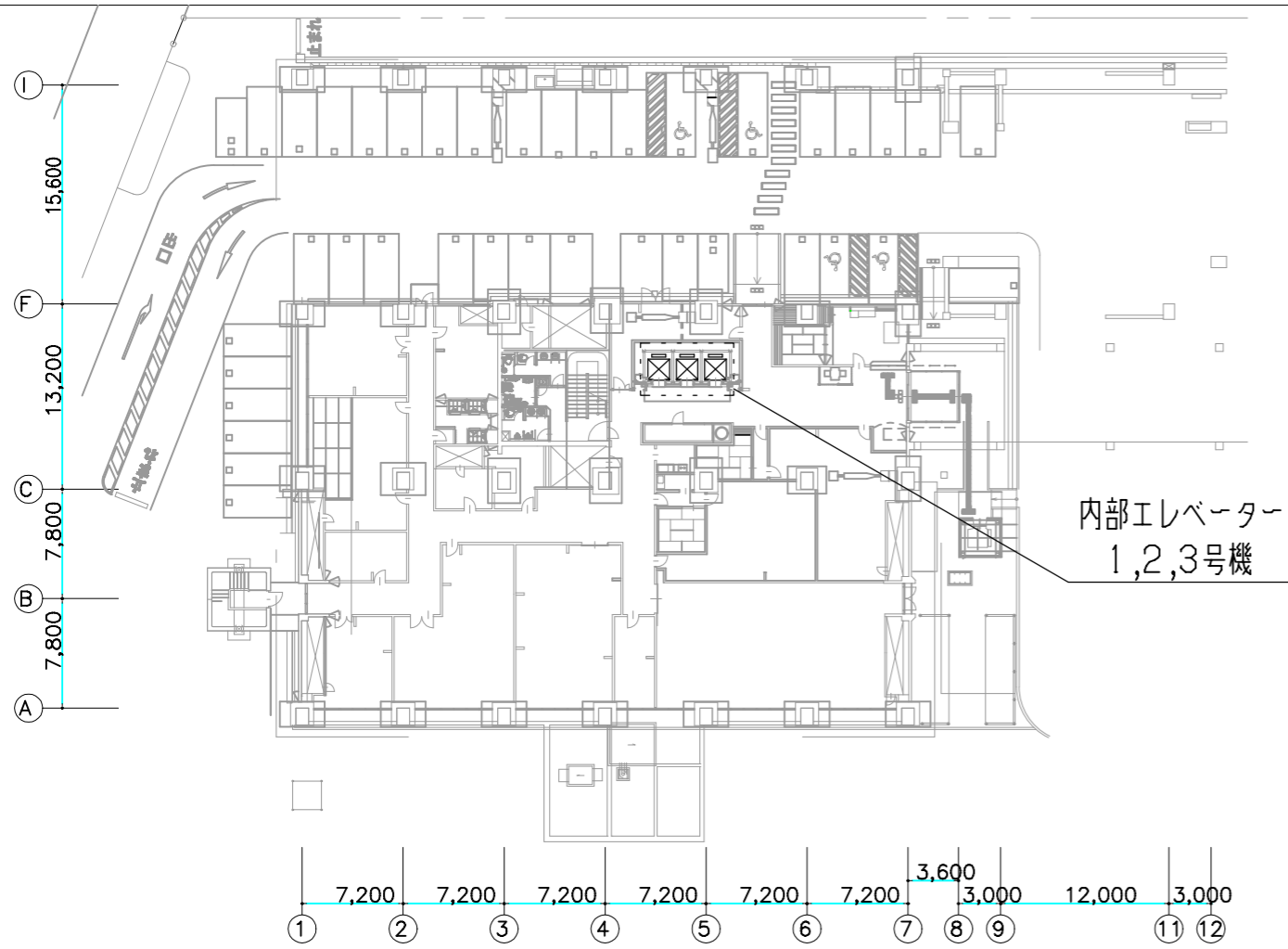
1階平面図 1/500
