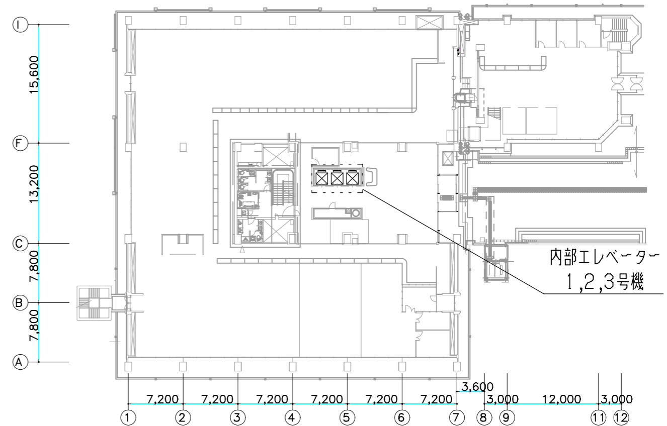
2階平面図 1/500
