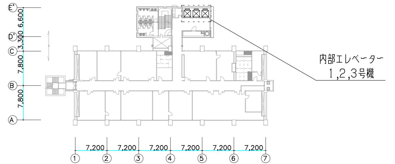
6階平面図 1/500
