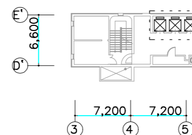
塔屋2階平面図 1/500
