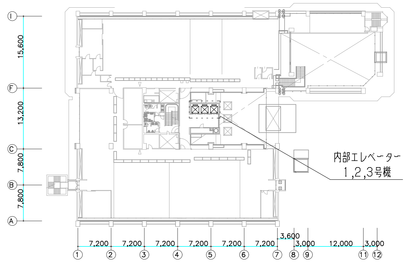
3階平面図 1/500
