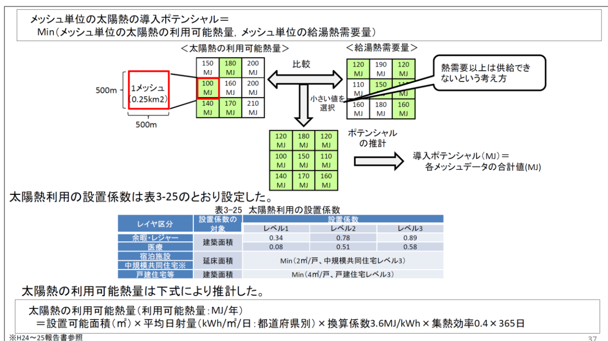
図10 REPOS における太陽熱導入ポテンシャルの算定方法
