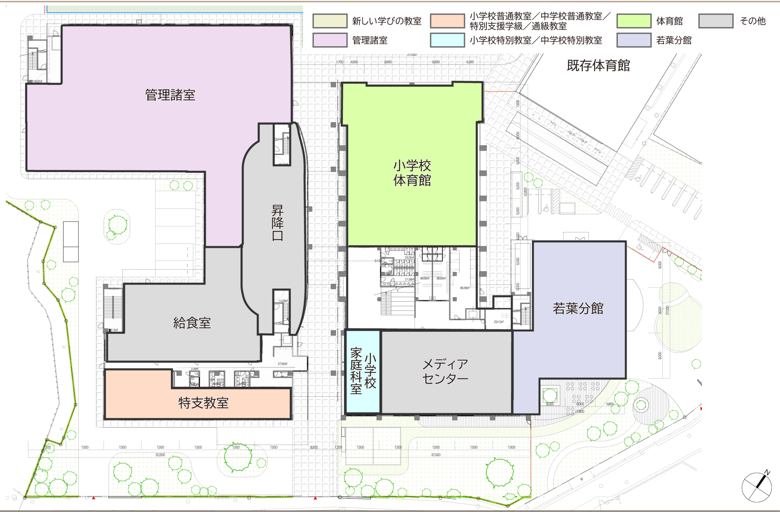
1 階 平面プラン
