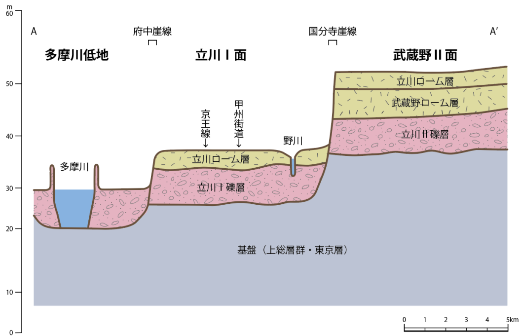
市域の地質断面図[上図のA-A'に対応] (「図説 調布の歴史」(調布市)をもとに作成)
