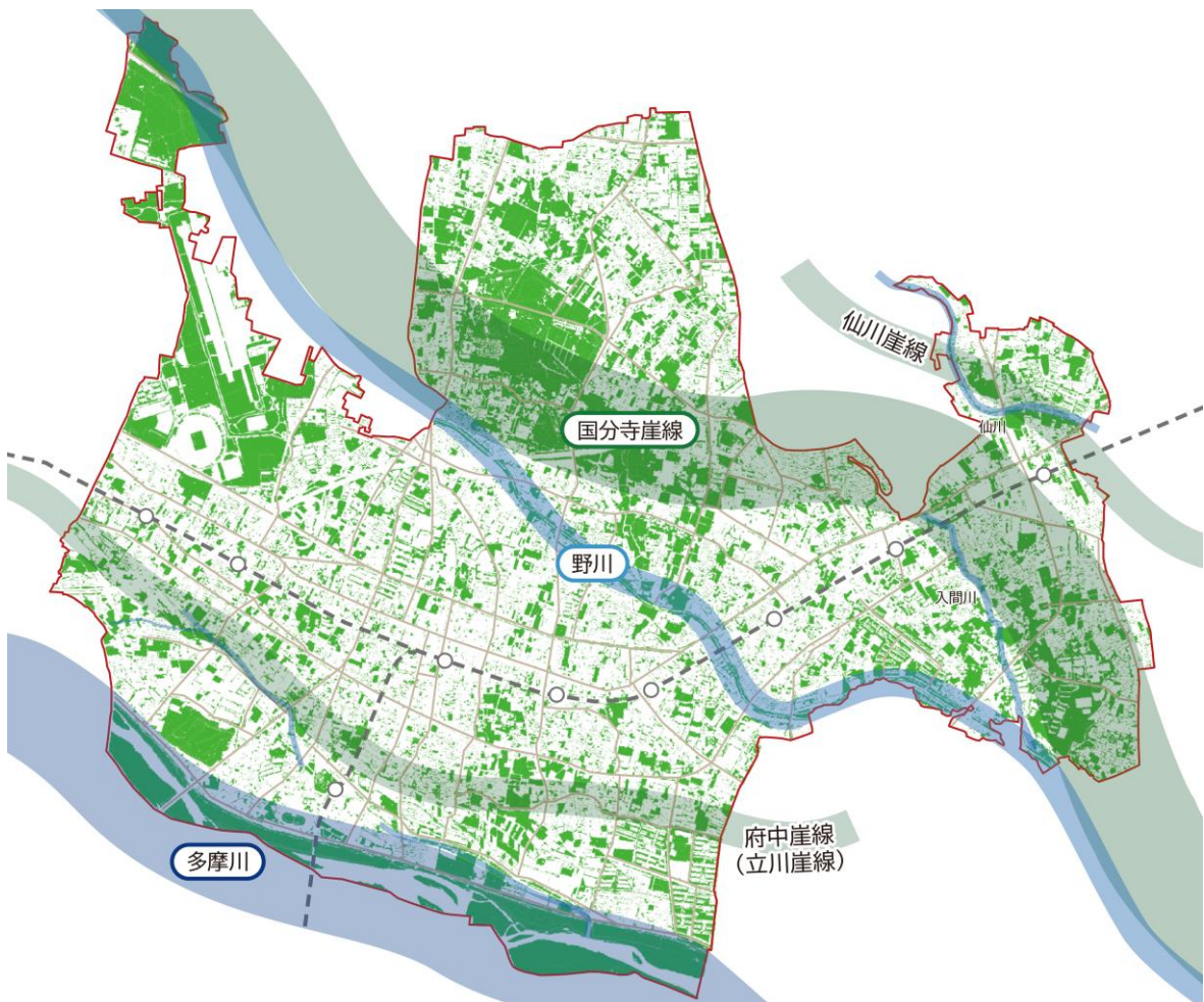
「地形変化が生み出す多様な景観」を示す景観構造(模式図)
