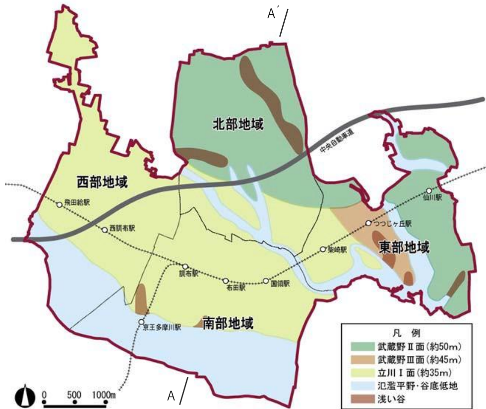
市の地形面区分 (「図説 調布の歴史」調布市)
