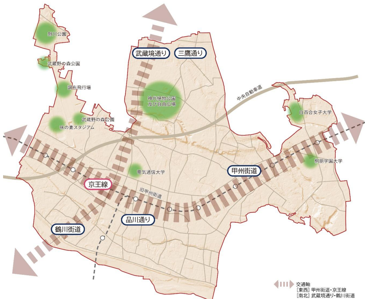
「街道沿いに発展したまちの成り立ちが作る景観」を示す景観構造(模式図)
