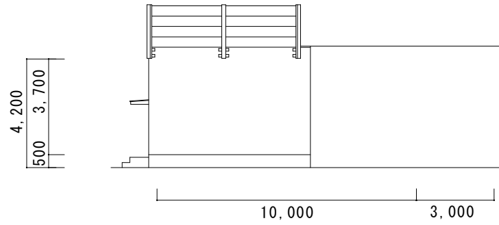
西側立面図（改修後）
