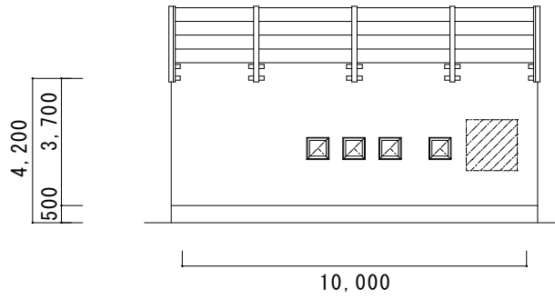
東側立面図（改修後）
