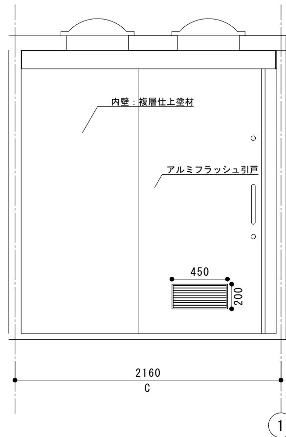
バリアフリースイレ 展開図 S=1:30
