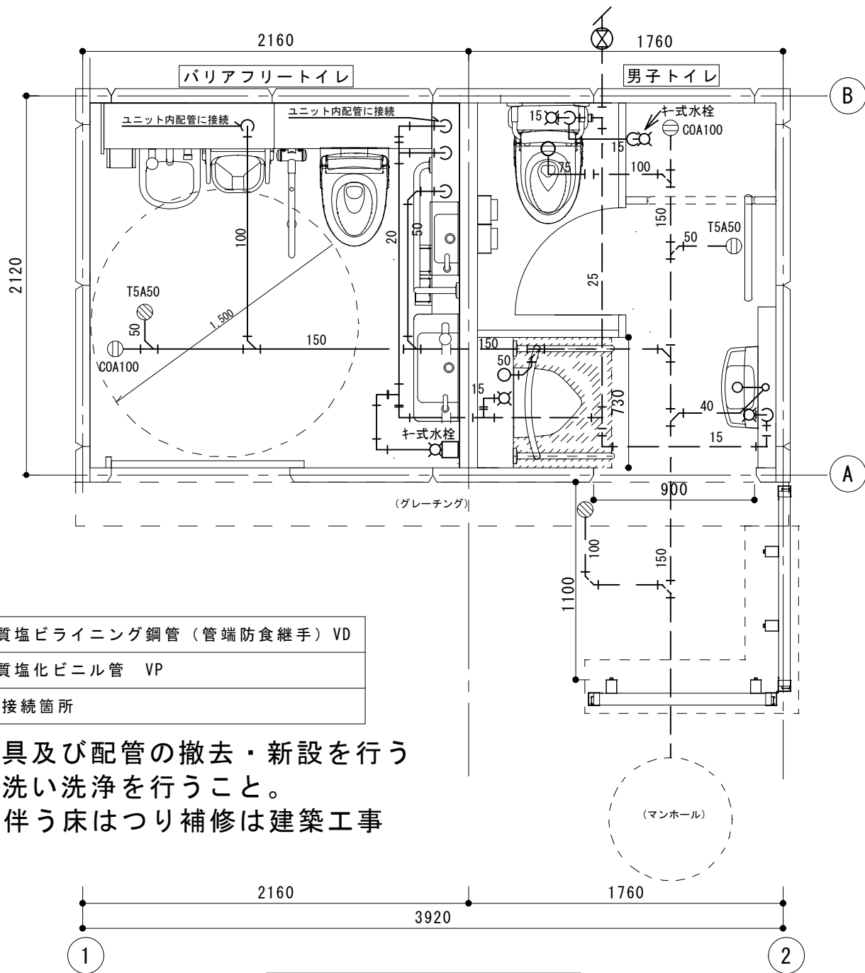
平面図（改修後） S=1：30
