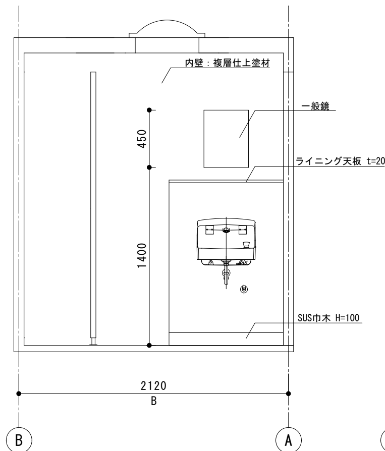
男子トイレ 展開図 S=1:30
