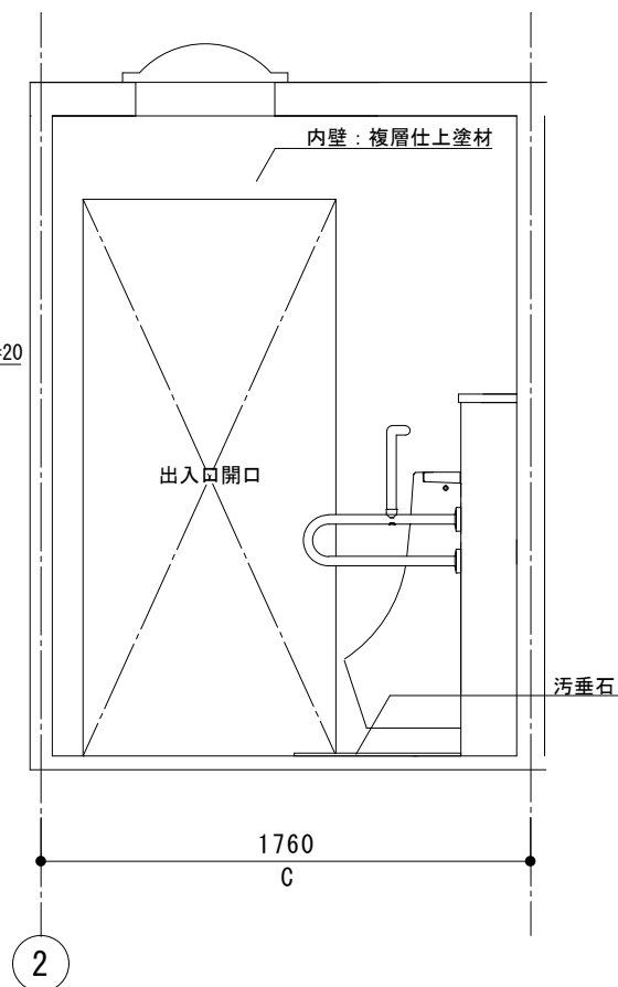
バリアフリースイレ 展開図 S=1:30
