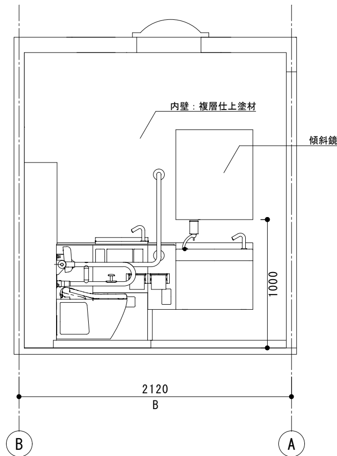
バリアフリースイレ 展開図 S=1:30
