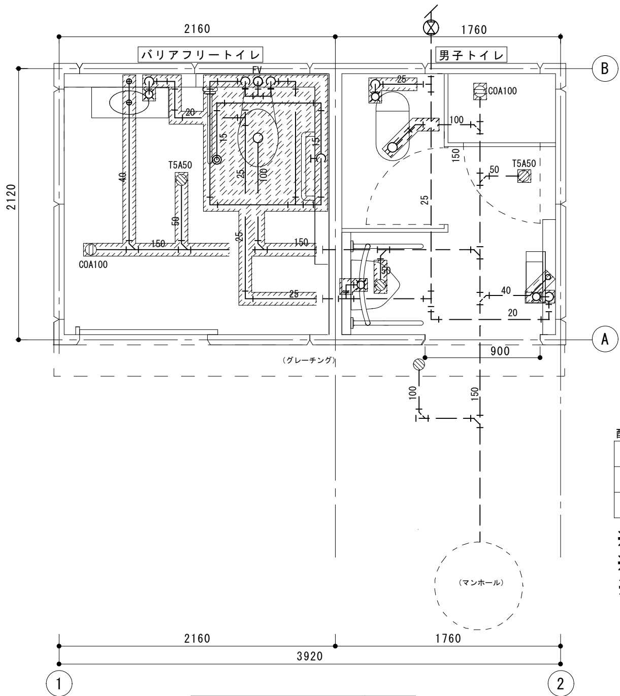
平面図（改修前） S=1：30
