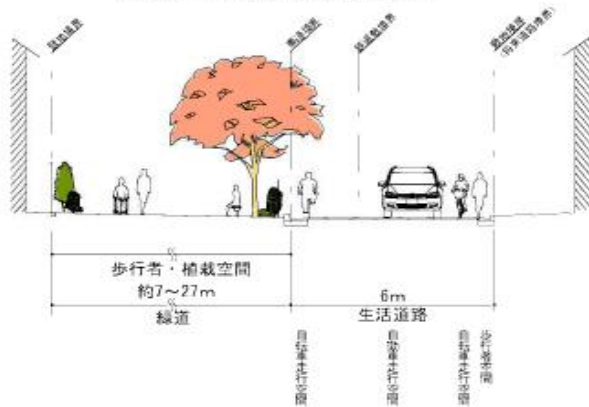
緑道、生活道路等標準断面
