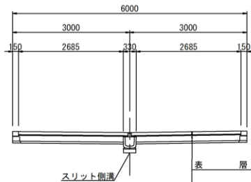
区画道路1号・3号 標準断面図
