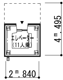
外部エレベーター1階平面図 1/200
