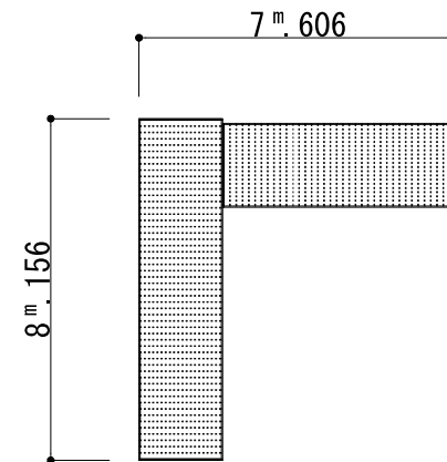
渡り廊下屋根伏図 1/200
