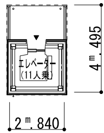
外部エレベーター2階平面図 1/200
