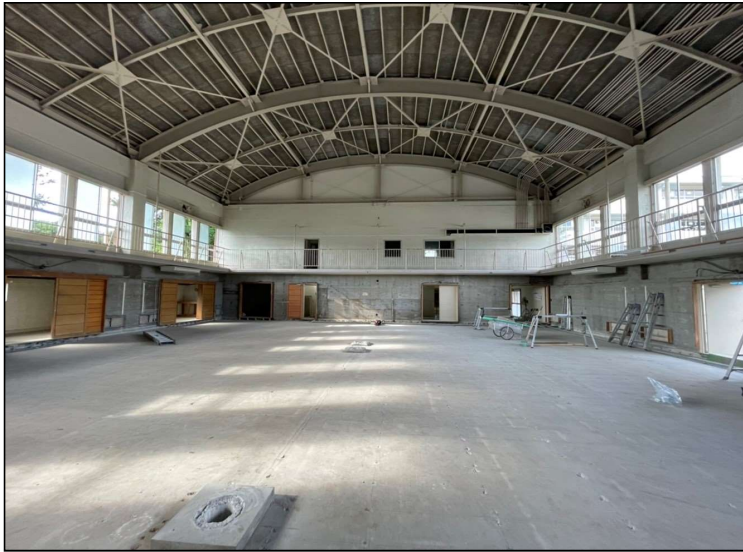
No.1 調布市立第一小学校体育館改修工事 体育館内部撤去 施工状況
