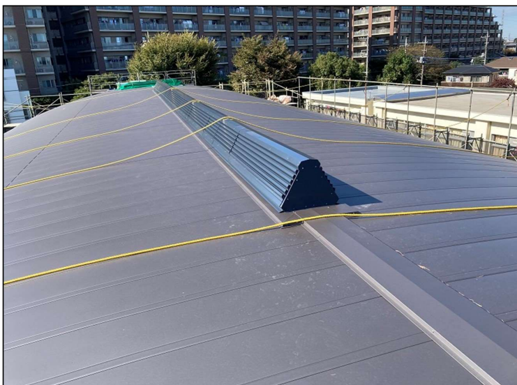
No.3 調布市立上ノ原小学校体育館外部改修工事 体育館屋根 施工状況
