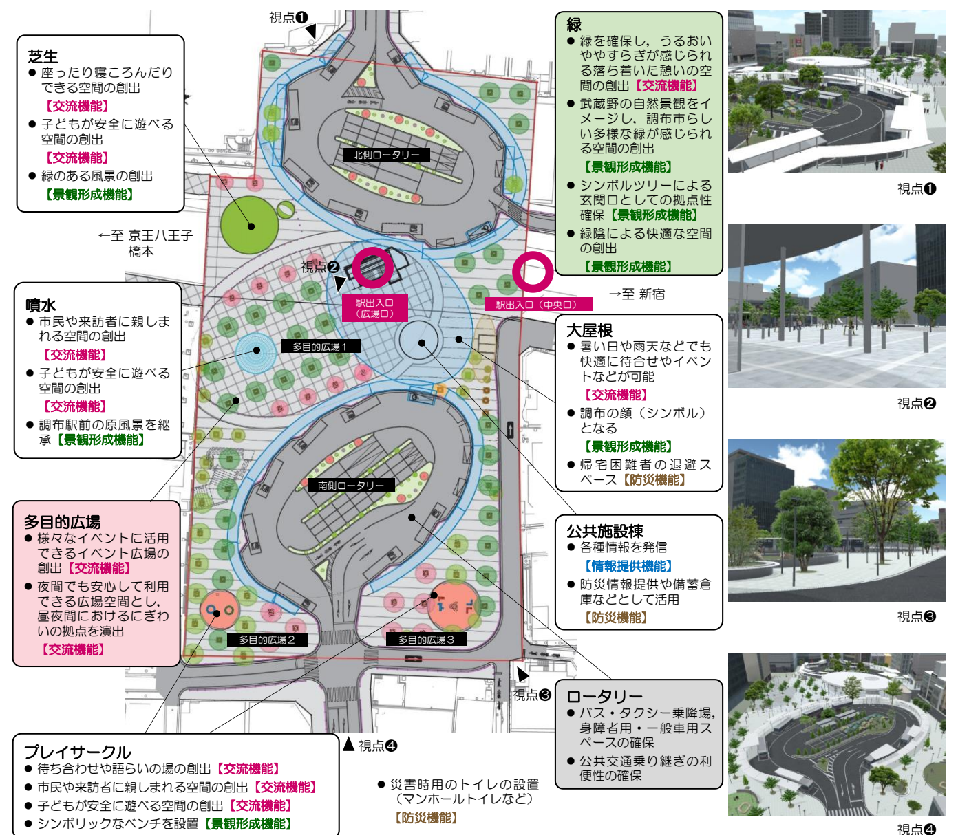
調布駅前広場検討図（平成25年7月）
