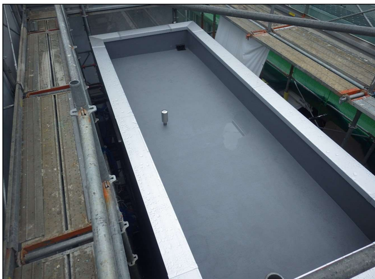
No.9 調布市東部公民館外部エレベーター設置ほか工事 屋上防水 施工状況
