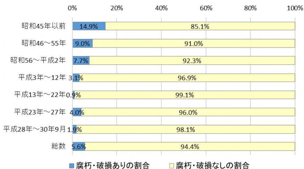
【建築時期別の老朽状況の割合】
